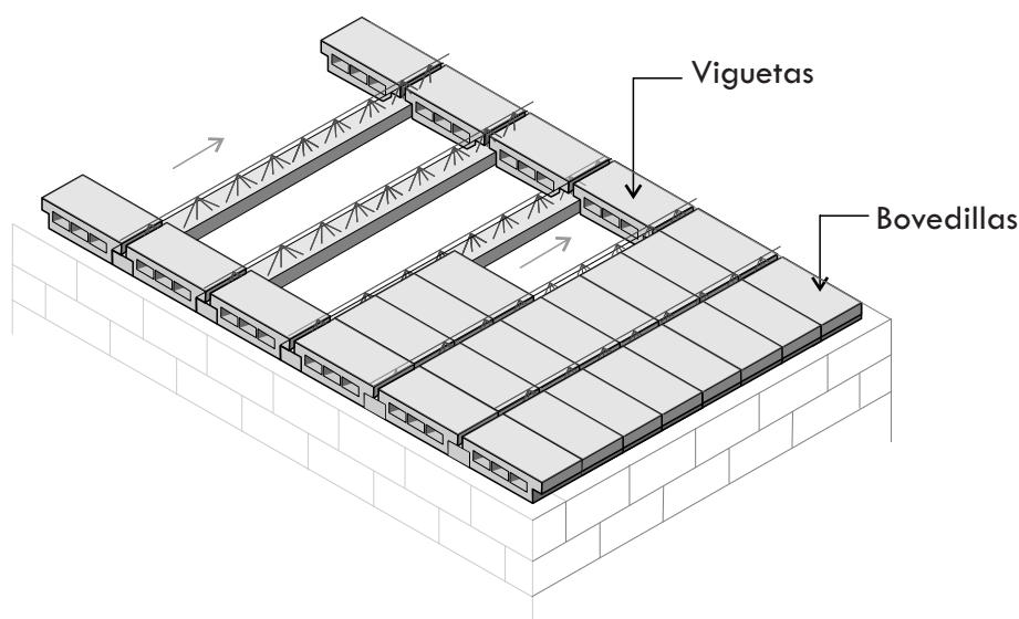
Figura 2 – Colocación de las Bovedillas No se ha dibujado el apuntalado
