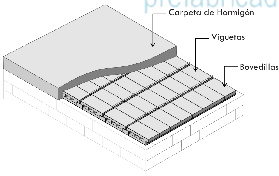
Figura 2 – Llenado de la carpeta de Compresión
