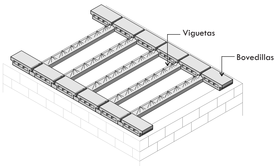
Figura 1 – Colocación de las Viguetas No se ha dibujado el apuntalado
