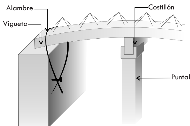
Figura 2 – Contraflecha Detalle de resolución
